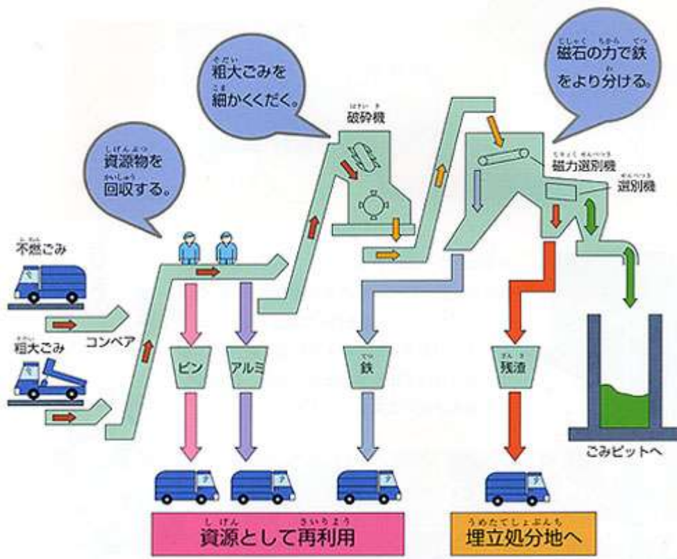
[参考] 破碎・選別処理フロー
