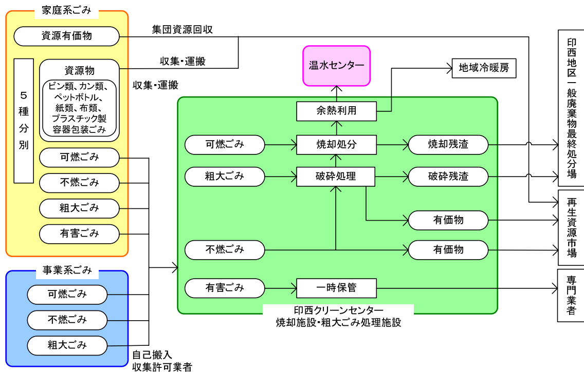
図 3.1 ごみ処理フロー
