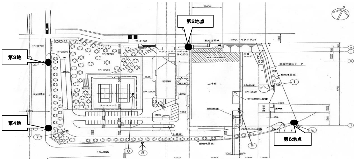
測定位置図
